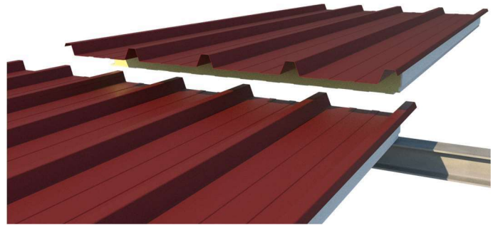
2. Sobald die erste Paneeelreihe fertiggestellt ist, das erste Paneeel überlappen.
