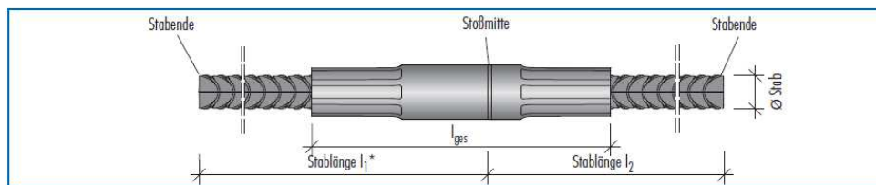
Teil A + B verschraubt, l_1 und l_2 = Stablänge für den Bewehrungsplan, *bei gebogenen Stäben die gestreckte Länge und das Biegemaß angeben
