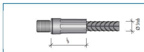
Muffenteil B
