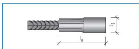
Muffenteil A
